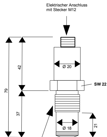
Prozessanschlussgewinde G 1/2"
