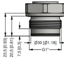
G1" DIN 3852 mit 2x O-Ring, SW41 p N ≤ 2 bar
