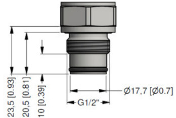
G1/2" DIN 3852 mit 2x O-Ring, SW27 p N ≥ 1 bar
