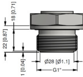
G1" DIN 3852 frontbündig, SW41
