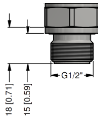
G1/2" DIN 3852 frontbündig, SW27 p N ≥ 1 bar
